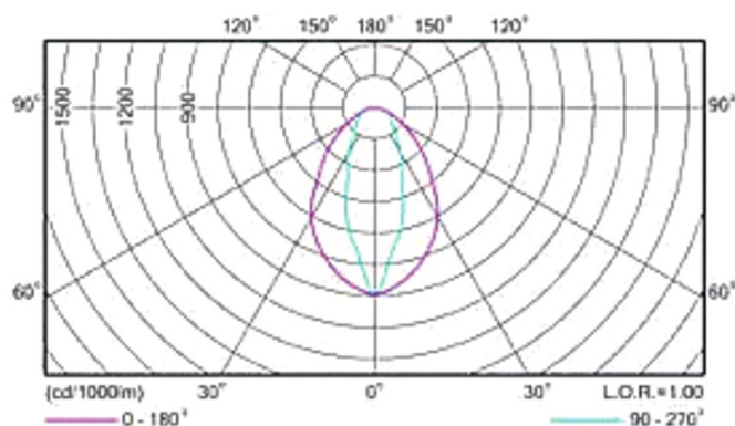
Диаграмма направленности
